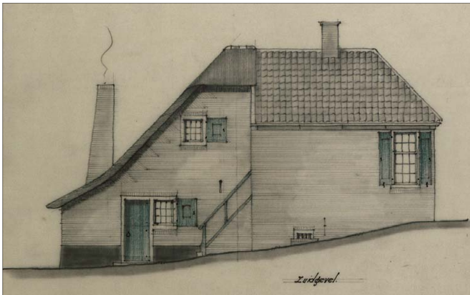
Tekening van het pand Wakkerendijk 170. Zicht op de zuiderzijgevel met links de toegang naar het woongedeelte en in het midden de trap naar de vroegere kleermakerij. Bouwtekening uit 1959, gemaakt i.v.m. de restauratie, door architect D. Verheus. (Collectie Rijksdienst Cultureel Erfgoed).
