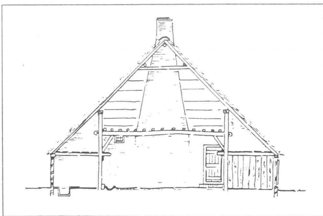
Dwarsdoorsnede boerderij met ankerbalkgebint
