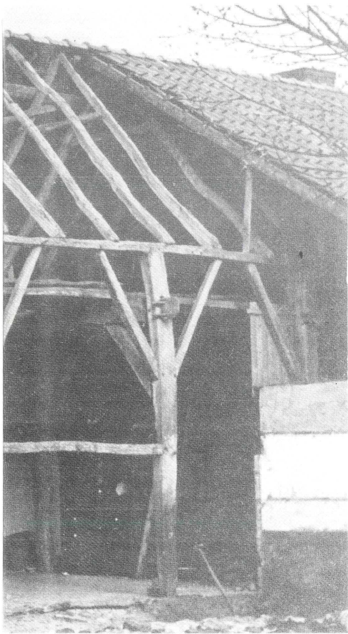
Gedeeltelijk ontmantelde boerderij met zicht op draagconstructie
