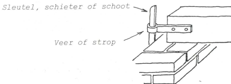
Balkenanker
