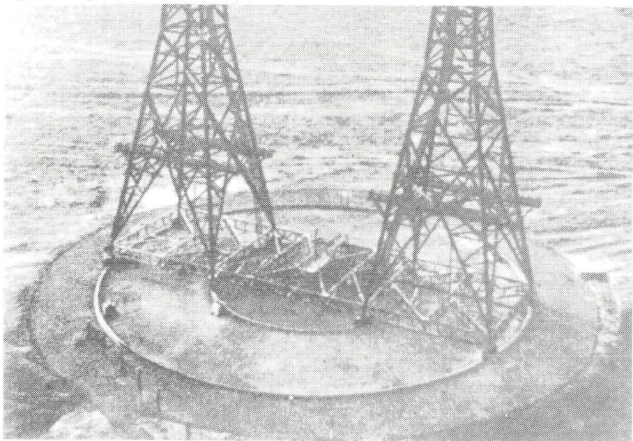
De twee antenne-masten op het draaibare onderstel. (Uit herinneringsalbum 'NSF')
