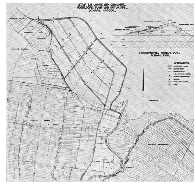
Situatiekaart behorend bij het voorlopig plan tot indijking van een gedeelte van het IJsselmeer ten oosten van de Meent en Gooise Maten.
